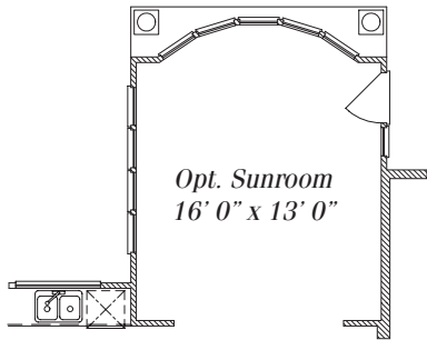
Optional Sunroom
